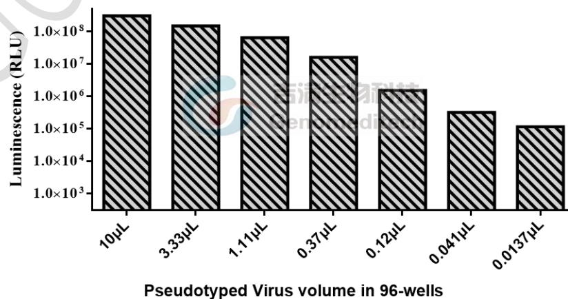
图2 吉满 SARS-CoV-2 Spike S 蛋白(Lambda)突变型假病毒感染 HEK293T-ACE2 测定 Luciferase 数值
